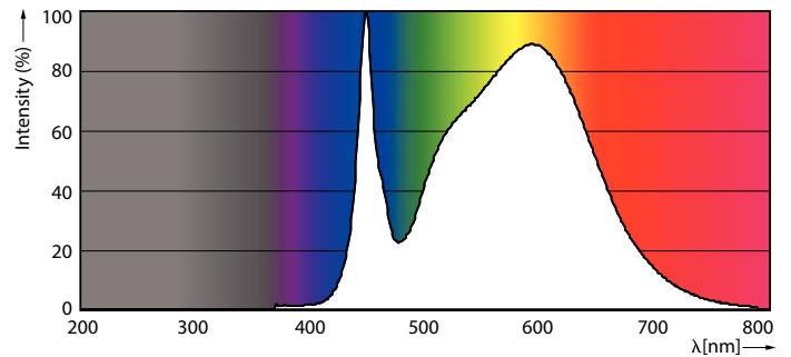
14W G13
