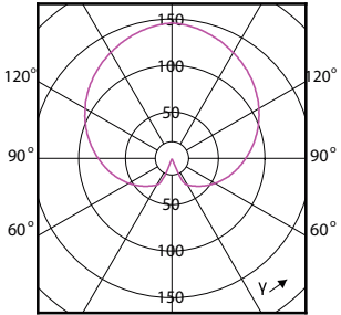
(cd/1000lm) 0°
