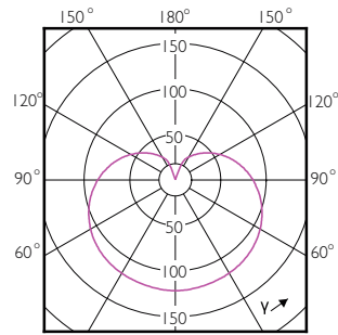
(cd/1000lm) 0° 150° 180° 150°
