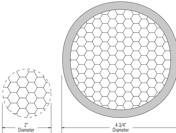
Cat. No. 7472 (Bare Edge Hex Cell Louver)
