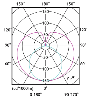
Light Distribution Diagram - Ledtube DE 600mm 9W 765 T8 G13
