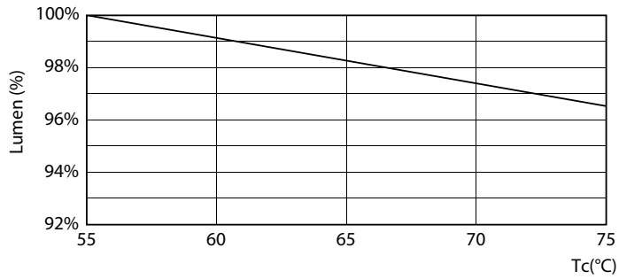
Lumen Maintenance Diagram - Ledtube DE 600mm 9W 740 T8 G13 RCA
