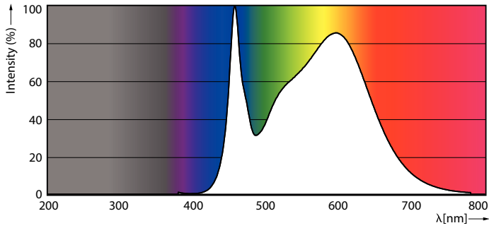
LEDtube COR 13,5W G13 1800lm 840
