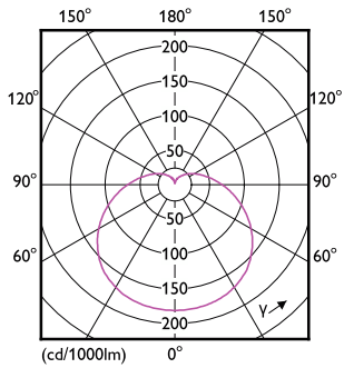
Light Distribution Diagram - 14A19/LED/865/FR/P/ND 2PF/6 NL
