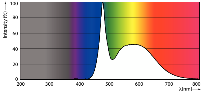
Spectral Power Distribution Colour - 14A19/LED/865/FR/P/ND 2PF/6 NL
