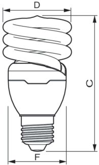
TORNADO 20W CDL E27 220-240V 1PF/6
