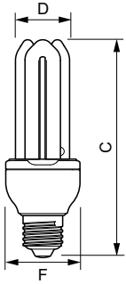
ECOHOME Stick 18W CDL E27 110-127V 1PF/6
