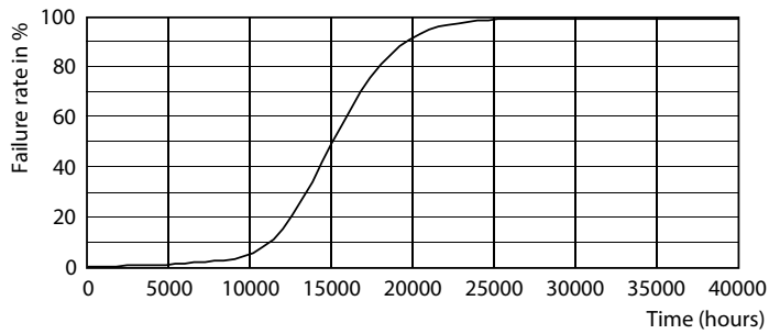
LEDtube G13
