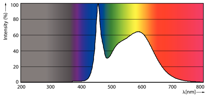
30W FA8
