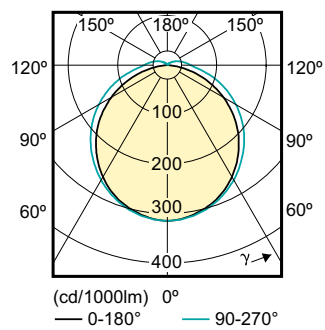
(cd/1000lm) 0° — 0-180° — 90-270°
