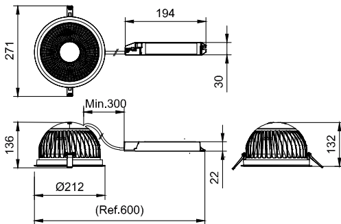
DN592B LED25/840 POE C D200 WH WB GM
