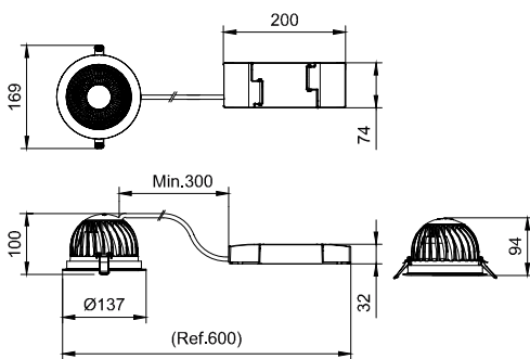
DN590B LED15/930 PSD C D125 WH MB GC
