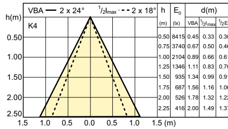
LDBE_CDM-Rm_20W_40D_0003-Beam diagram
