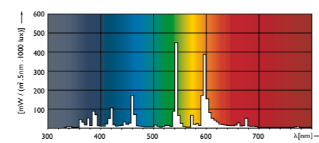
Master HPI-T Plus -400Вт
