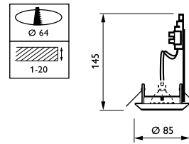
QBS570
