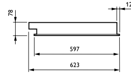
TBSI47 (2x36W)
