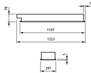
TBSI47 (2x36W)
