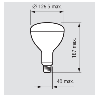
MLR 160 W E27
